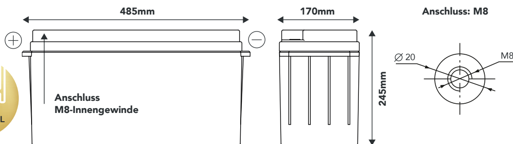
Abmaße: Länge 485mm | Breite 170mm | Höhe 245mm
