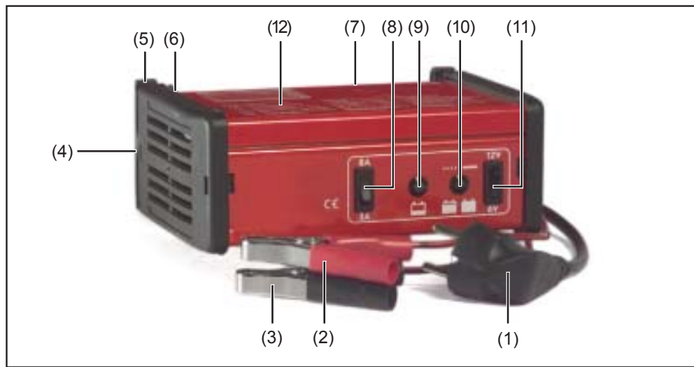
Abb.1 Bedienelemente und Anschlüsse
