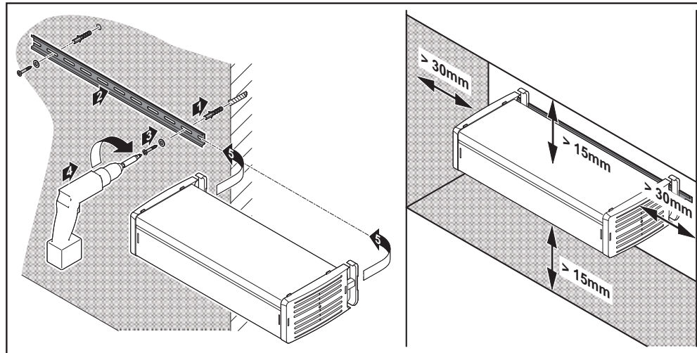
Afb. 2 Laadapparaat met de als extra verkrijgbare muursteun (rail TS 35, EN 50022) Afb. 3 Minimale afstanden
