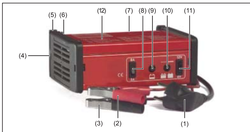
Afb. 1 Bedieningselementen en aansluitingen (symbolische foto)
